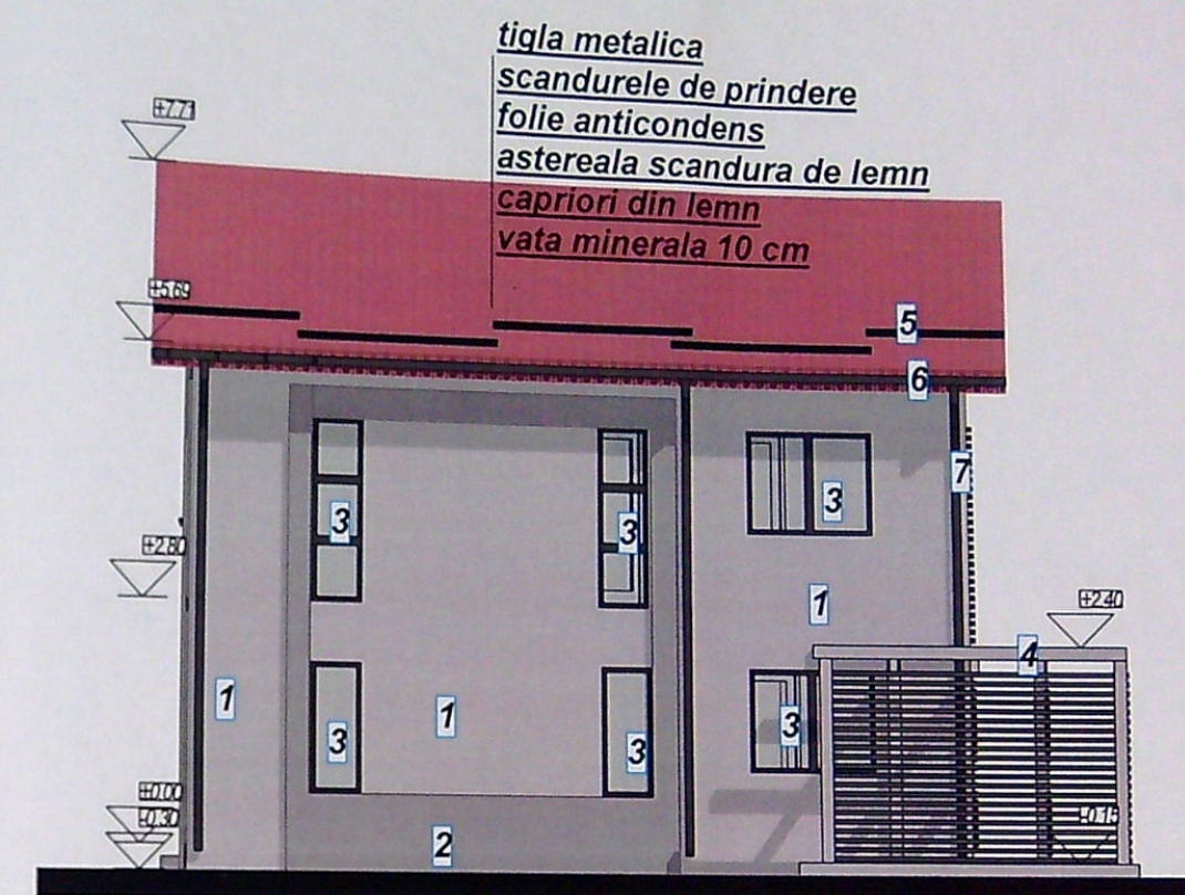
FATADA LATERALA DREAPTA(DE SUD)
