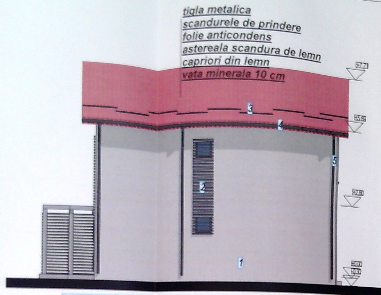
FATADA LATERALA STANGA(DE NORD)
